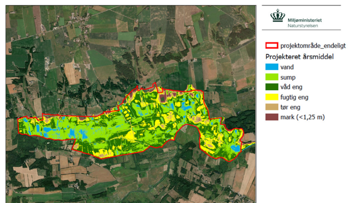
Figur 2: Oversigtskort over Kvorning lavbundsprojekt med arealernes forventede afvanding efter etablering af projektet.
